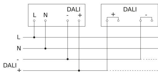
Diagrama electrónico interconexión DALI-2 APC con DALI-2 IPD
